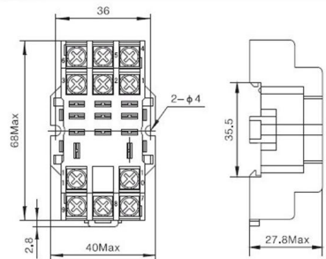
安装尺寸内部端子连接图
