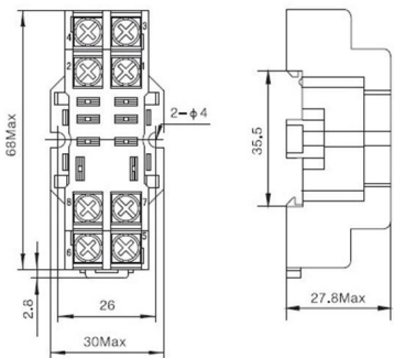
安装尺寸内部端子连接图
