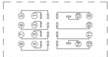
安装尺寸内部端子连接图
