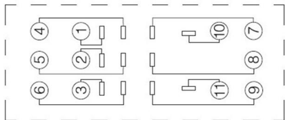
安装尺寸内部端子连接图
