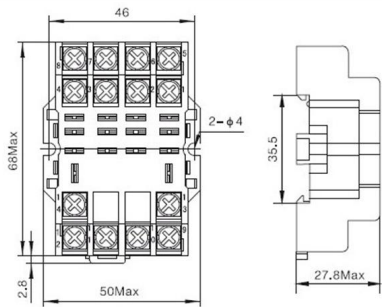
安装尺寸内部端子连接图
