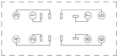
安装尺寸内部端子连接图
